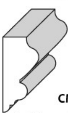
CMK 467 1-1/16" x 1-7/16"
